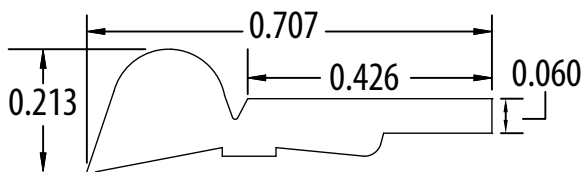
PN0484332 TFW-N4 Wiper
